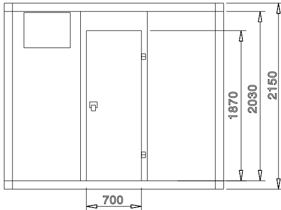
Zij aanzicht
